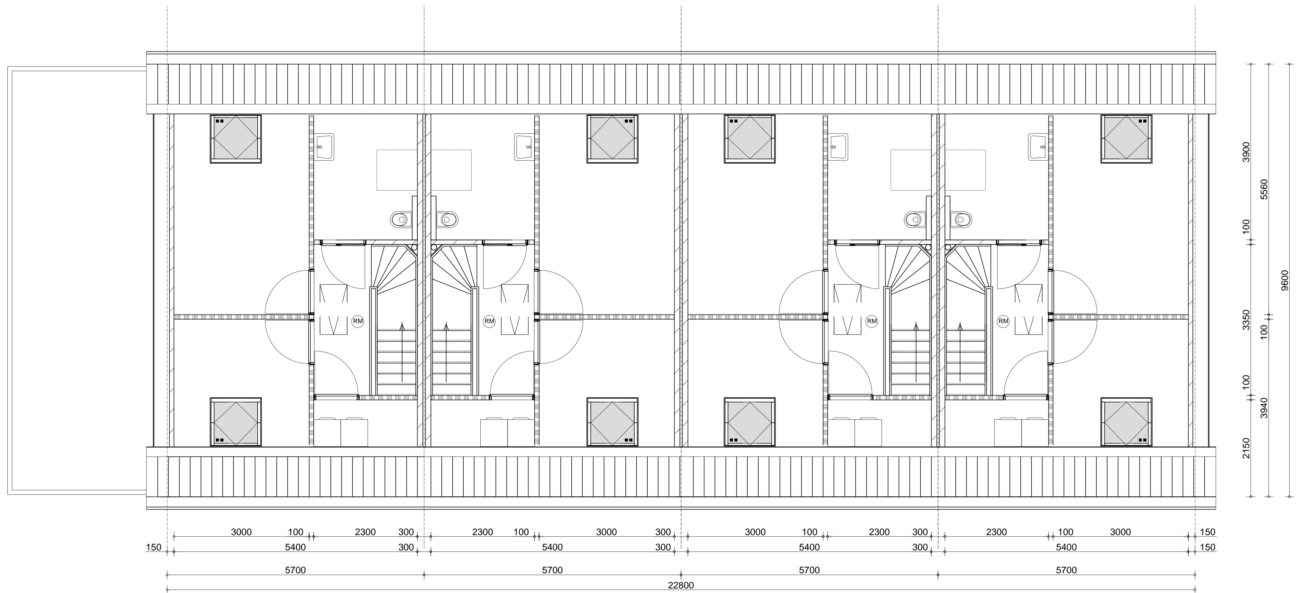
Verdieping 1:50
