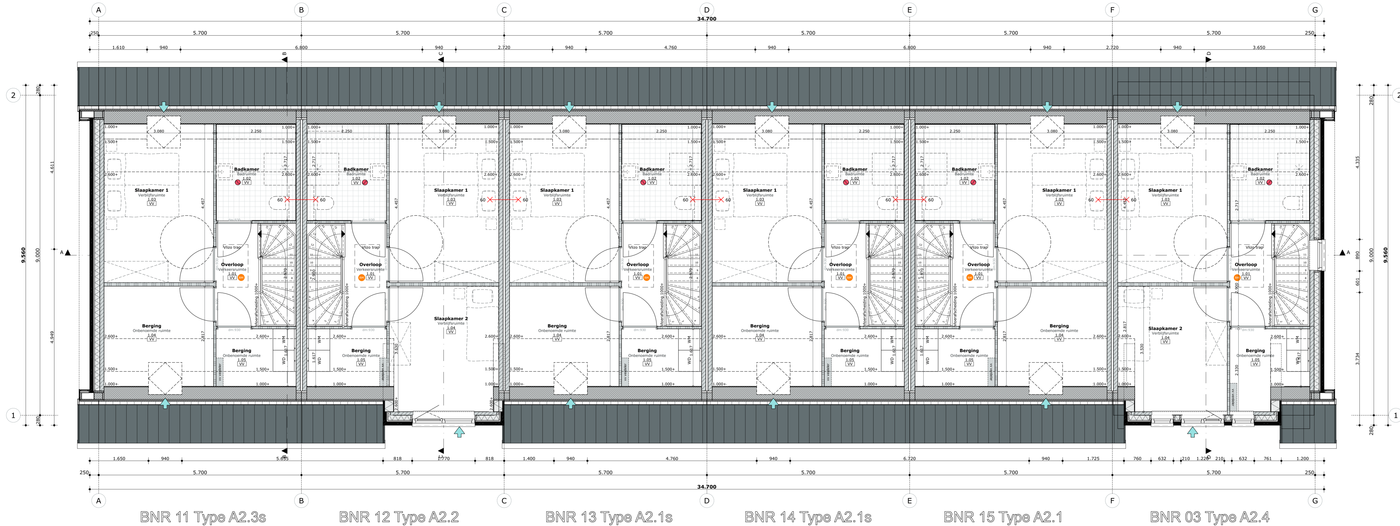
01 eerste verdieping
