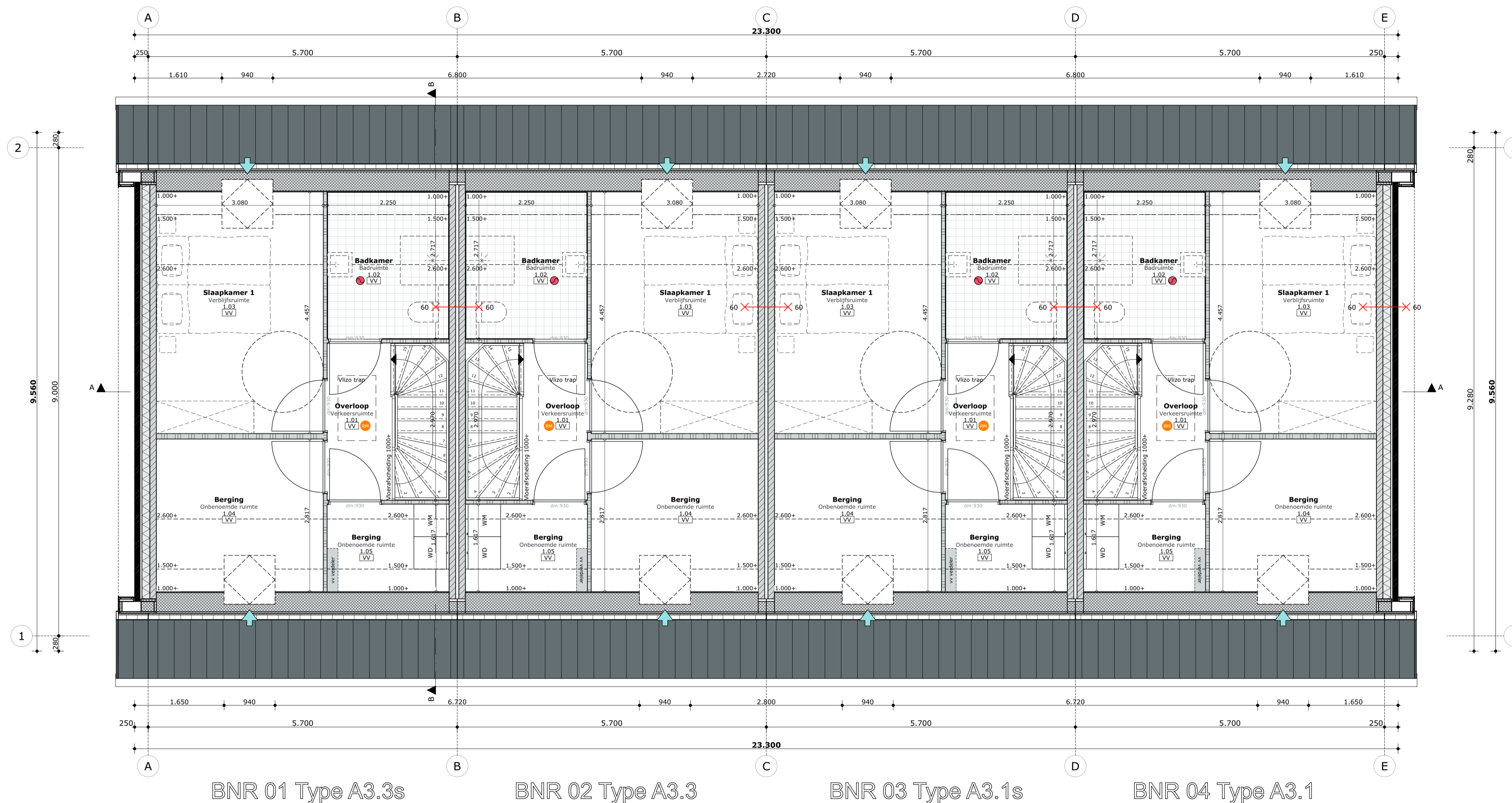
01 eerste verdieping
