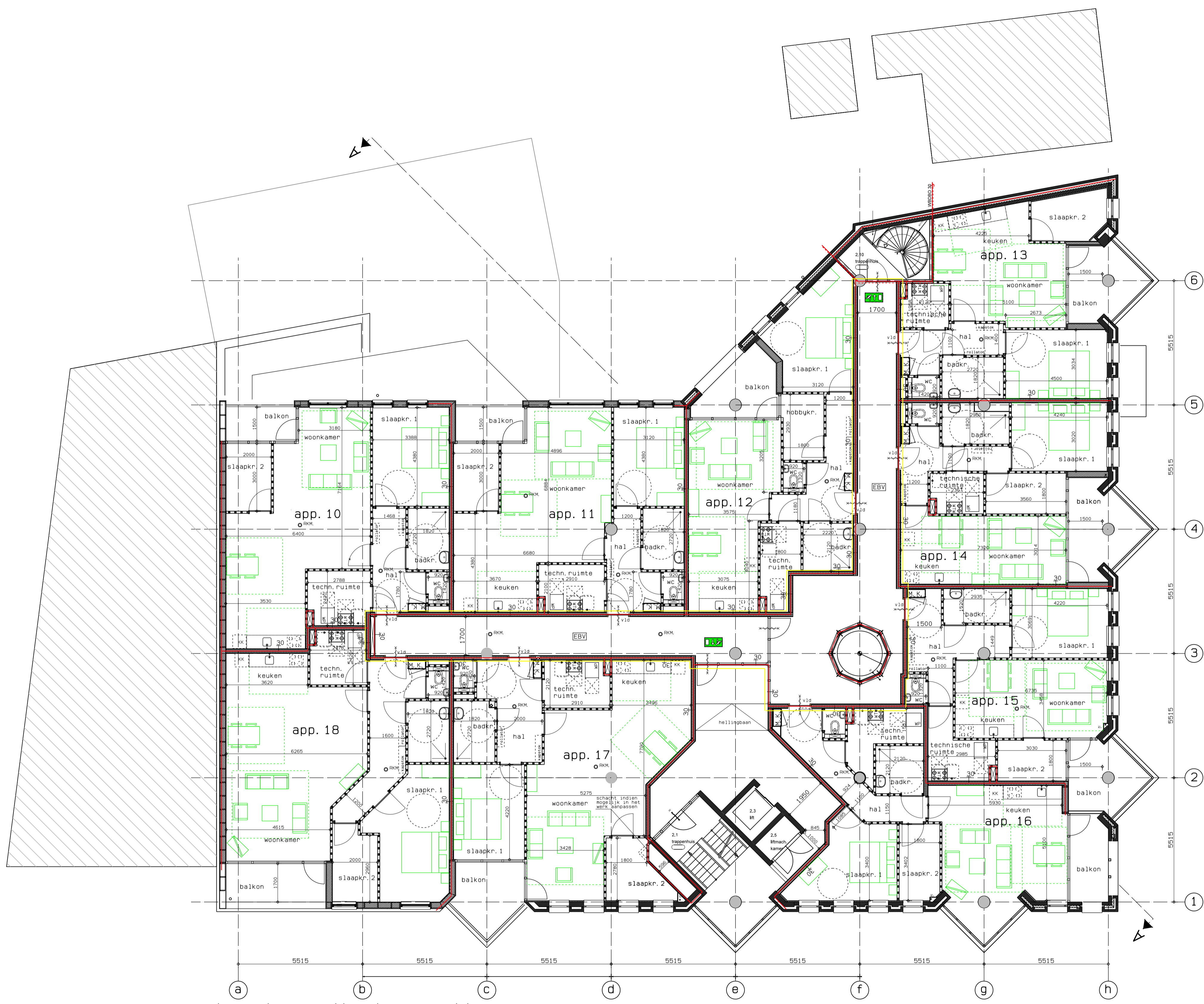
tweede verdieping gewijz.
